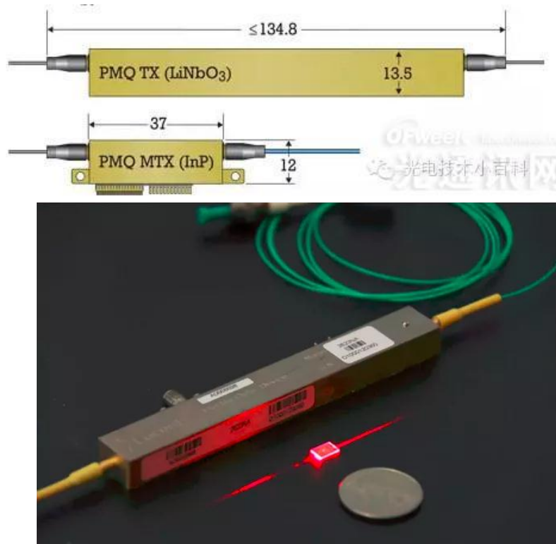
图：薄膜铌酸锂技术突破引领下一代光器件
