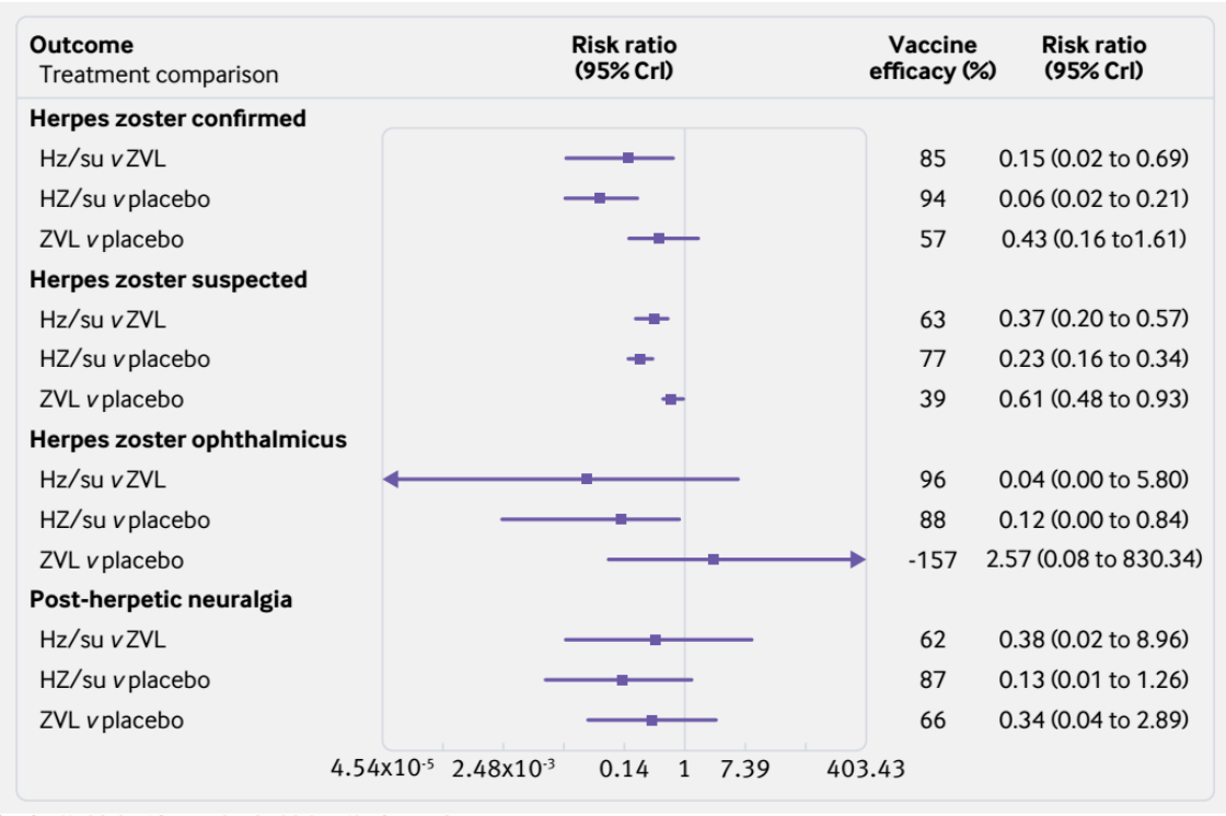
Meta分析Shingrix和Zostavax有效性对比
