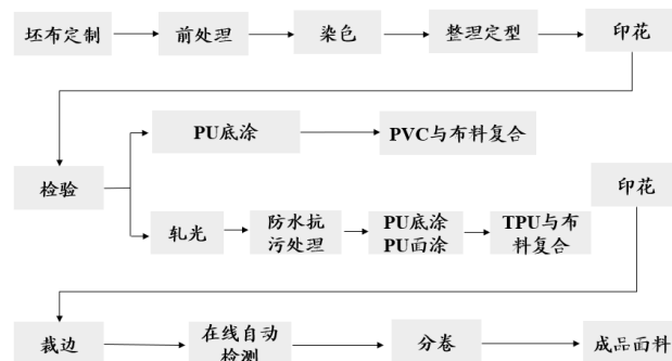
图 4：面料制作工艺流程
