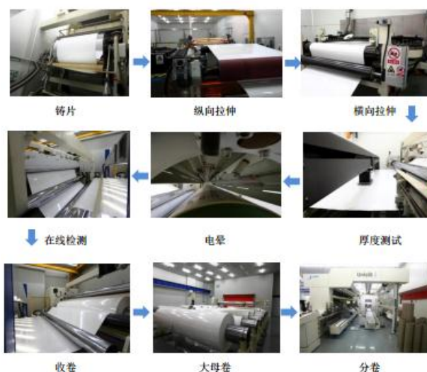
图 1 光学基膜与非涂布反射膜基本生产工艺图
