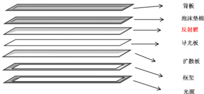
图9 LED 面板灯结构图
