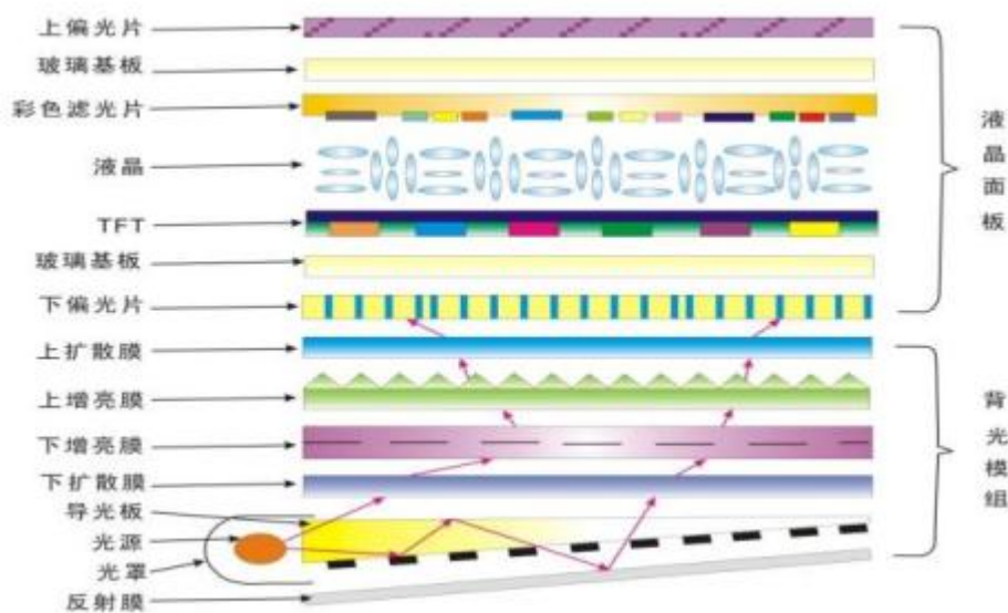
图8 液晶模组结构
