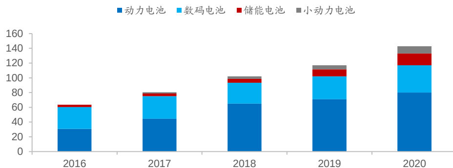
图 13: 2016-2020年中国各终端锂电池出货量 (GWh)
