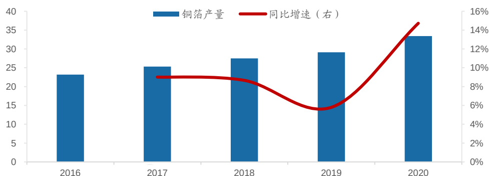
图 18：2016-2020年中国PCB铜箔产量（万吨）
