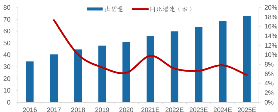
图 16：2016-2025全球PCB铜箔出货量及预测（万吨，%）
