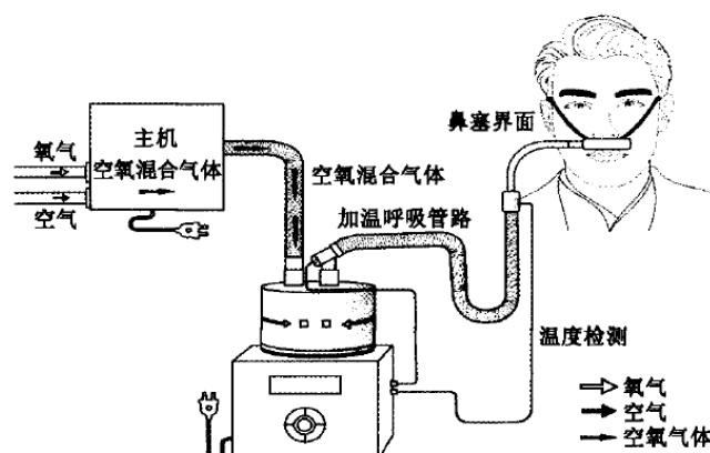
图18: 经鼻高流量湿化氧疗仪示意图
