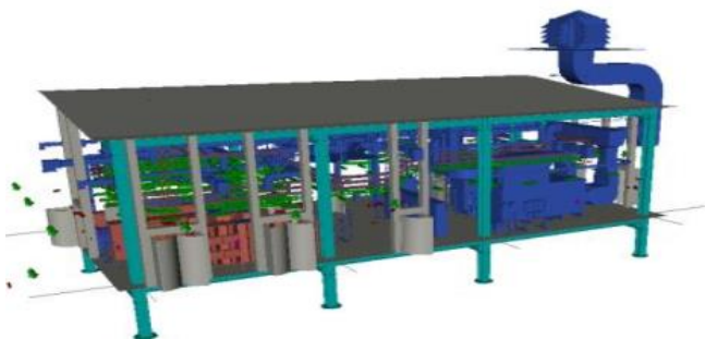
图表 24：电气模块
