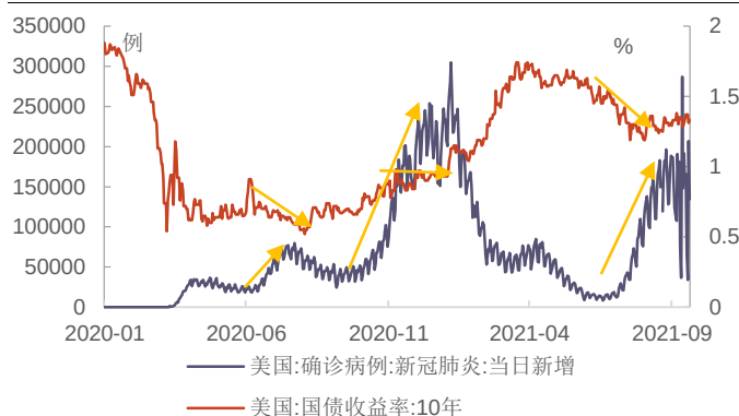
图 3：新冠新增病例大幅增加时，美债收益率受到一定的压力
