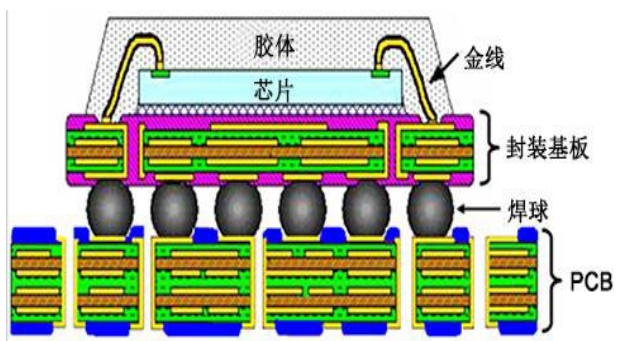
图表 15 封装基板示意图
