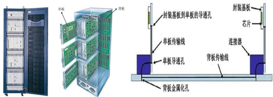
图表 12 背板与单板及其组装
