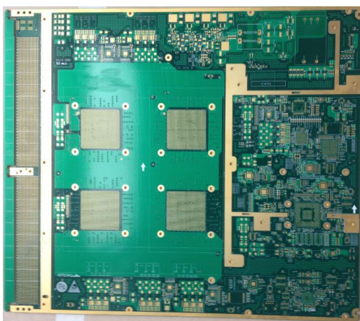
图表 13 100G 通信骨干网传输用高速系统板
