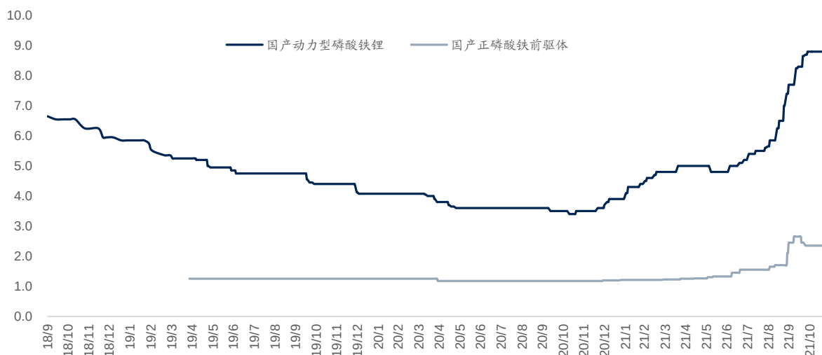
图 4: 磷酸铁、磷酸铁锂价格走势 (单位: 万元/吨)
