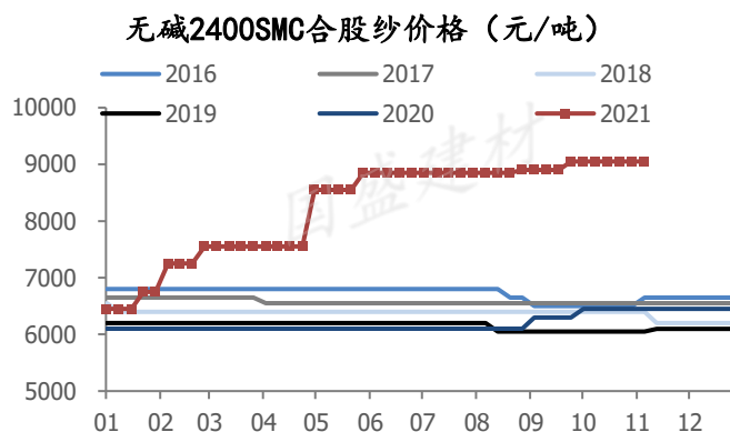
图表 81: 无碱 SMC 合股纱价格延续上行的趋势
