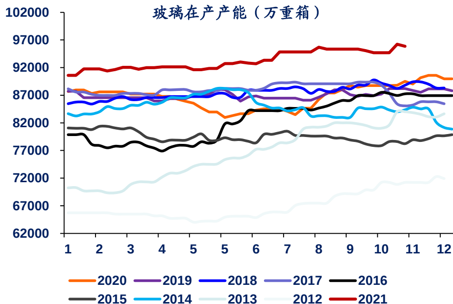
图19 玻璃在产产能回升至近年来高位水平
