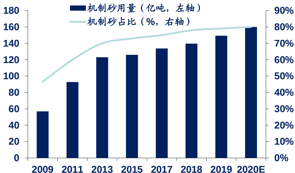
图12 机制砂用量及占比持续提升
