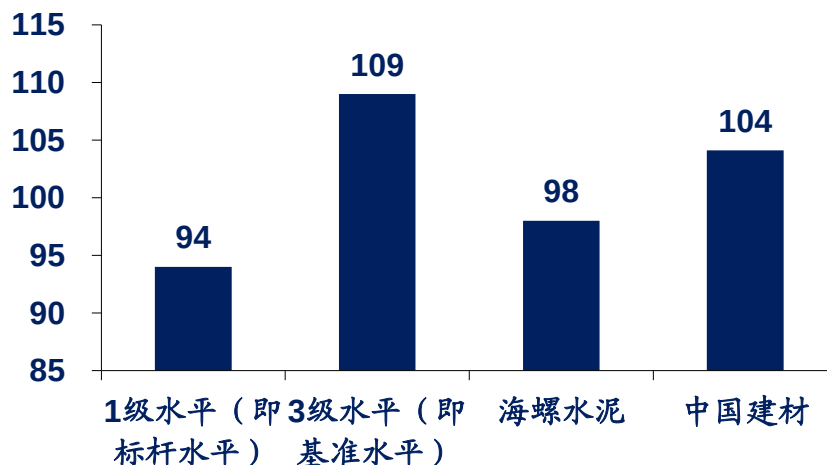
图3 龙头企业可比熟料综合煤耗和行业标准对比（kgce/t）
