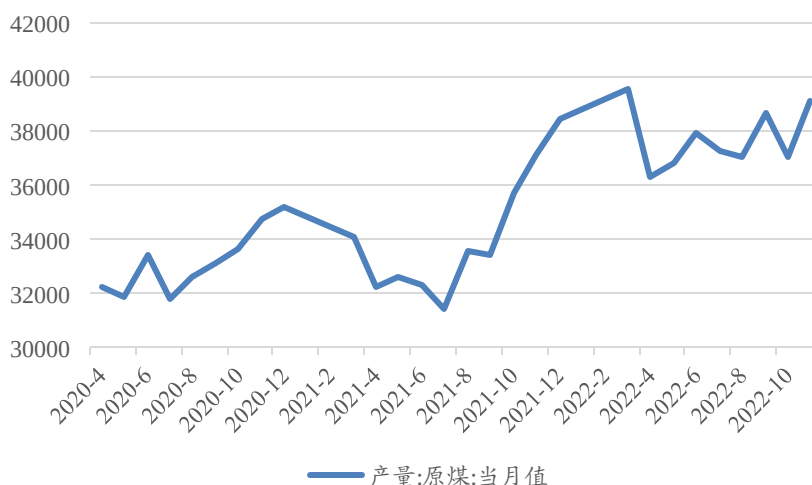
图 13 2022 年原煤产量整体呈震荡走势（单位：万吨）
