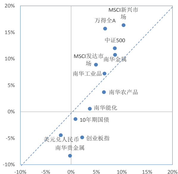
图 13：信用脉冲 12M 变化由正转负后资产平均回报
