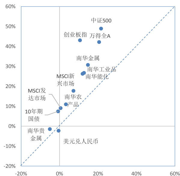
图 14：信用脉冲 12M 变化由负转正后资产平均回报
