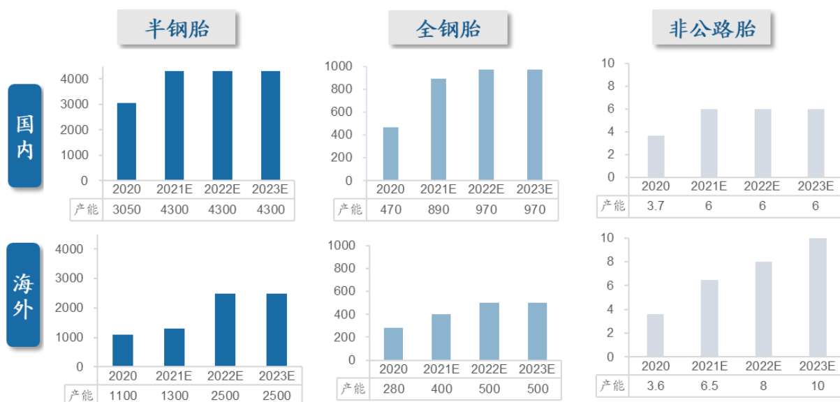
图6：赛轮轮胎国内外产能情况（半钢胎、全钢胎单位为万条/年，非公路胎单位为万吨/年）
