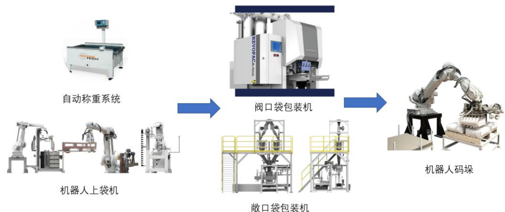
图表 19 自动化工业纸袋包装流程示意图
