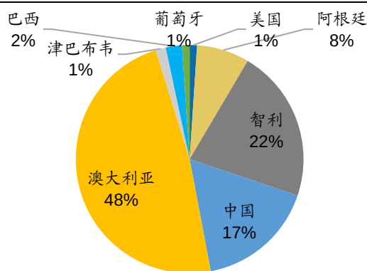
图 3：2020 年全球锂资源产量分布结构
