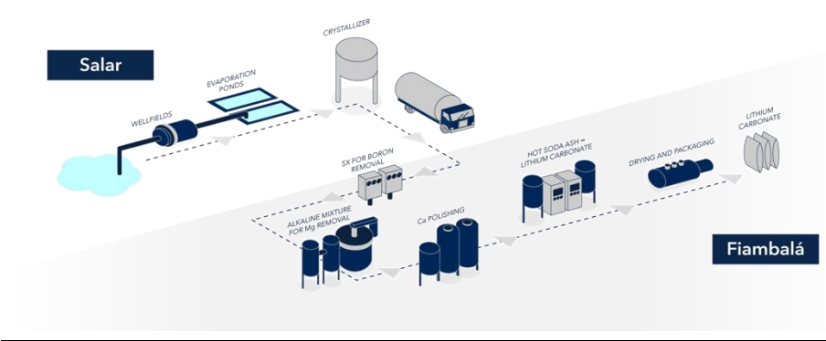
图 22：3Q 项目设备流程图
