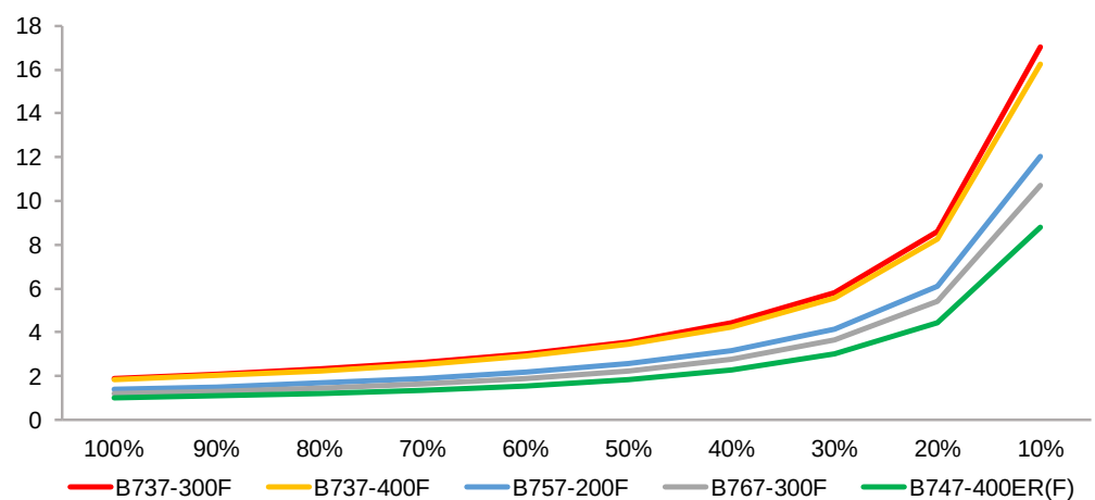
图表 73 不同载运率下不同机型的吨公里成本比较图
