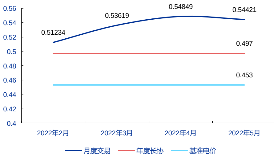
图6：广东省2022年电价情况（元/千瓦时，含税）
