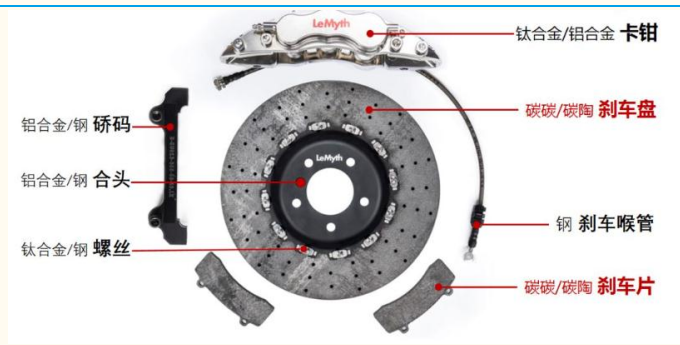
图表 28：汽车刹车制动盘的零部件构成
