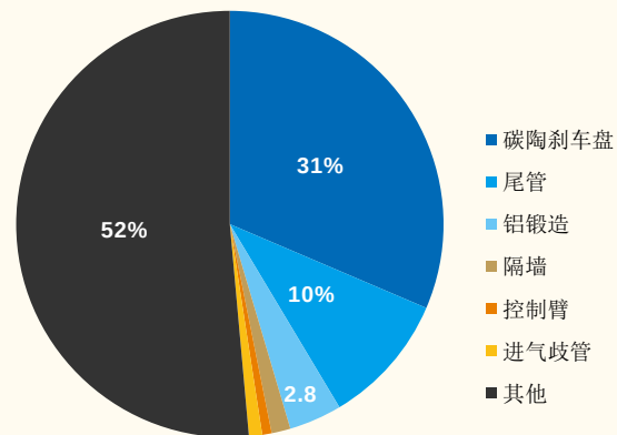
图表 30：丰田雷克萨斯 RCF 跑车各环节减重占比
