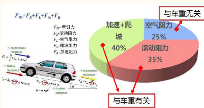
图表 31：汽车行驶中 75%的阻力与车重相关
