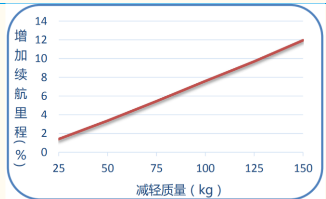
图表 32：汽车续航里程与汽车质量呈现负相关
