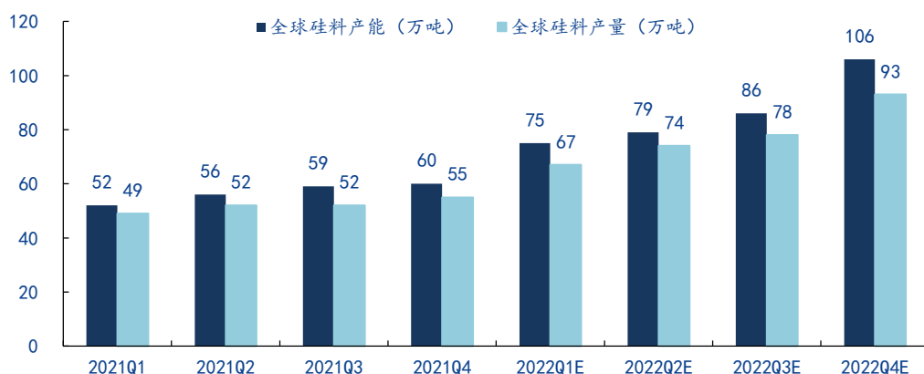
图表 21 2021-2022 硅料产能及产量变化
