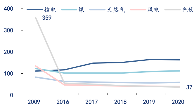
图表 16 不同发电方式度电成本（单位：美元/MWh）
