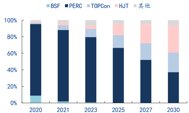
图表 26 电池技术路线变化
