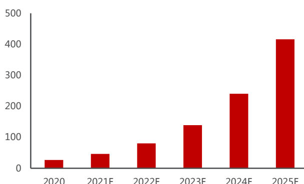
图 18：全球储能市场装机量预测（GWh）
