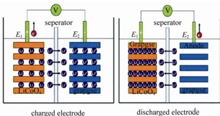
图 9：锂离子电池充放电原理图
