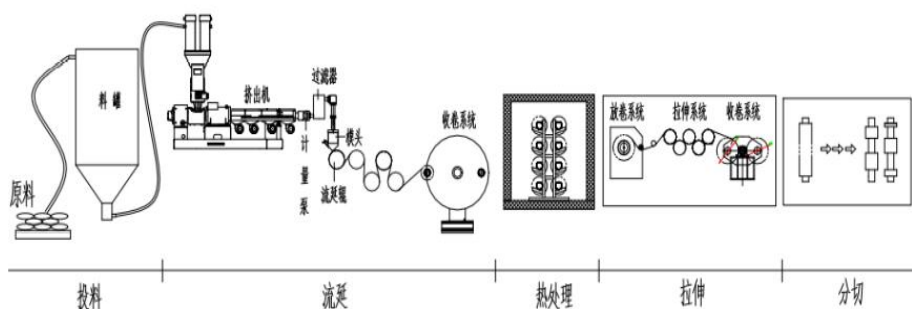
图 11：干法单拉隔膜工艺流程
