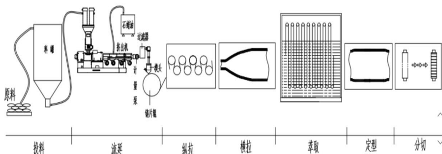
图 12：湿法隔膜工艺流程
