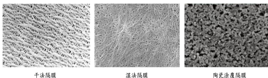
图 10：干法、湿法与涂覆隔膜的微观表征图
