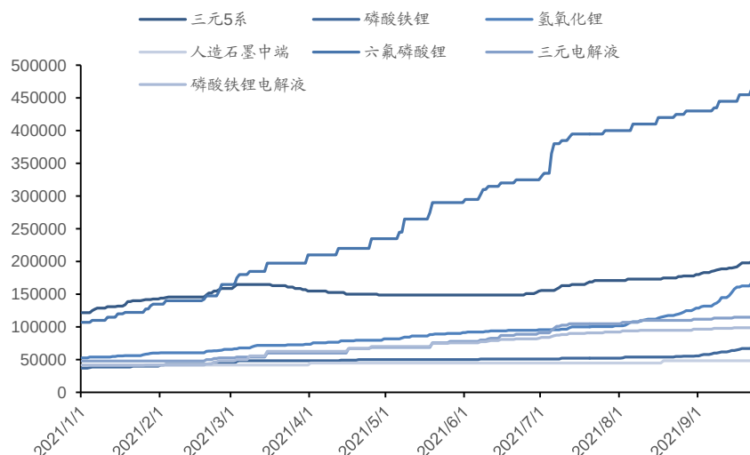
图 24：锂电主材价格情况（元/吨）
