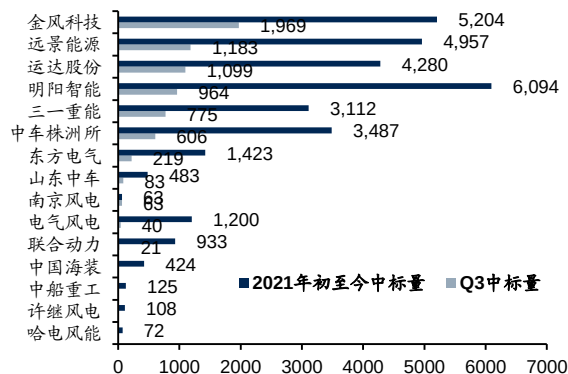
图 52: 各风机厂商中标容量 (MW)
