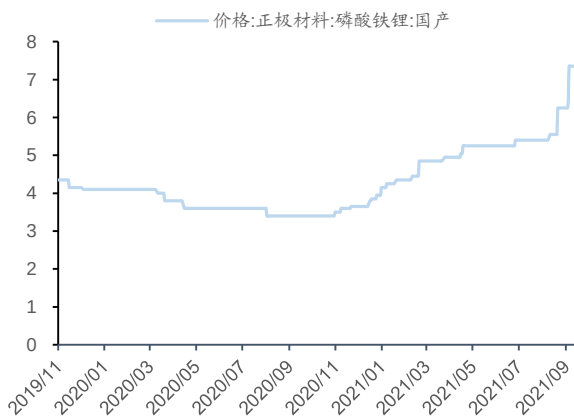
图 27: 正极磷酸铁锂市场价格一览 (万元/吨)
