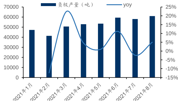
图 21: 国内负极材料产量 (吨)
