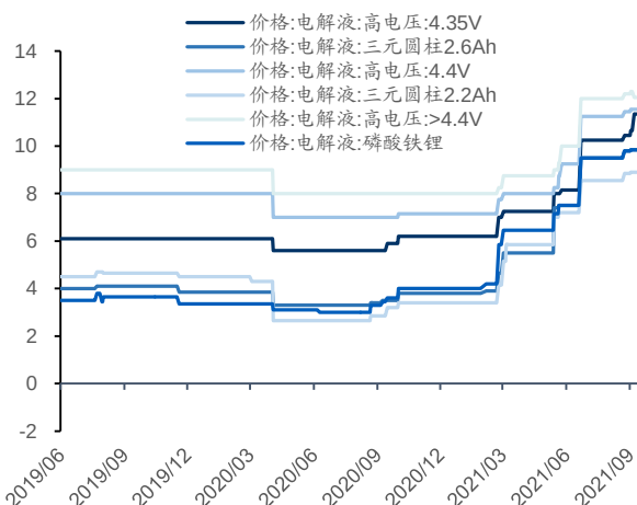
图 31: 电解液市场价格一览 (万元/吨)
