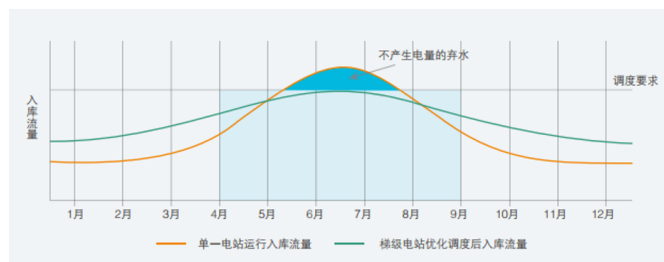
图44：梯级联调效应减少弃水
