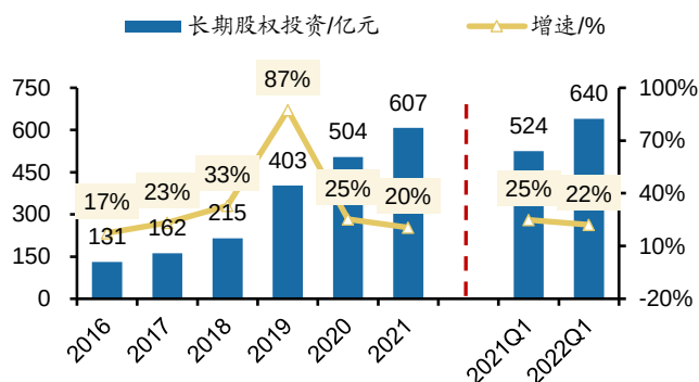
图49: 2016-2021年长期股权投资CAGR达35.9%
