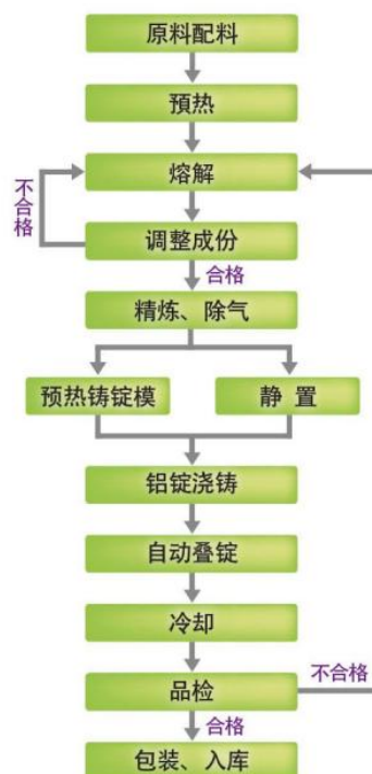
图表32： 怡球资源铝合金锭熔炼铸造工艺流程图
