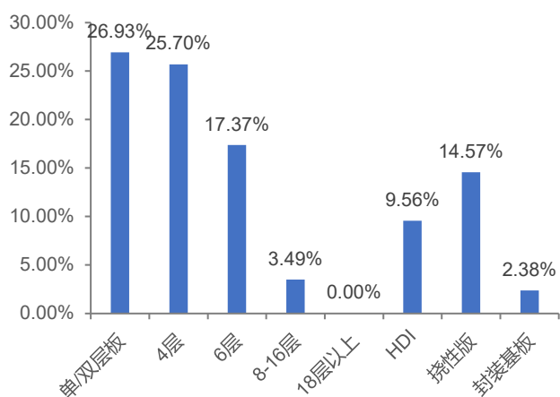
图表 11 汽车电子 PCB 需求结构
