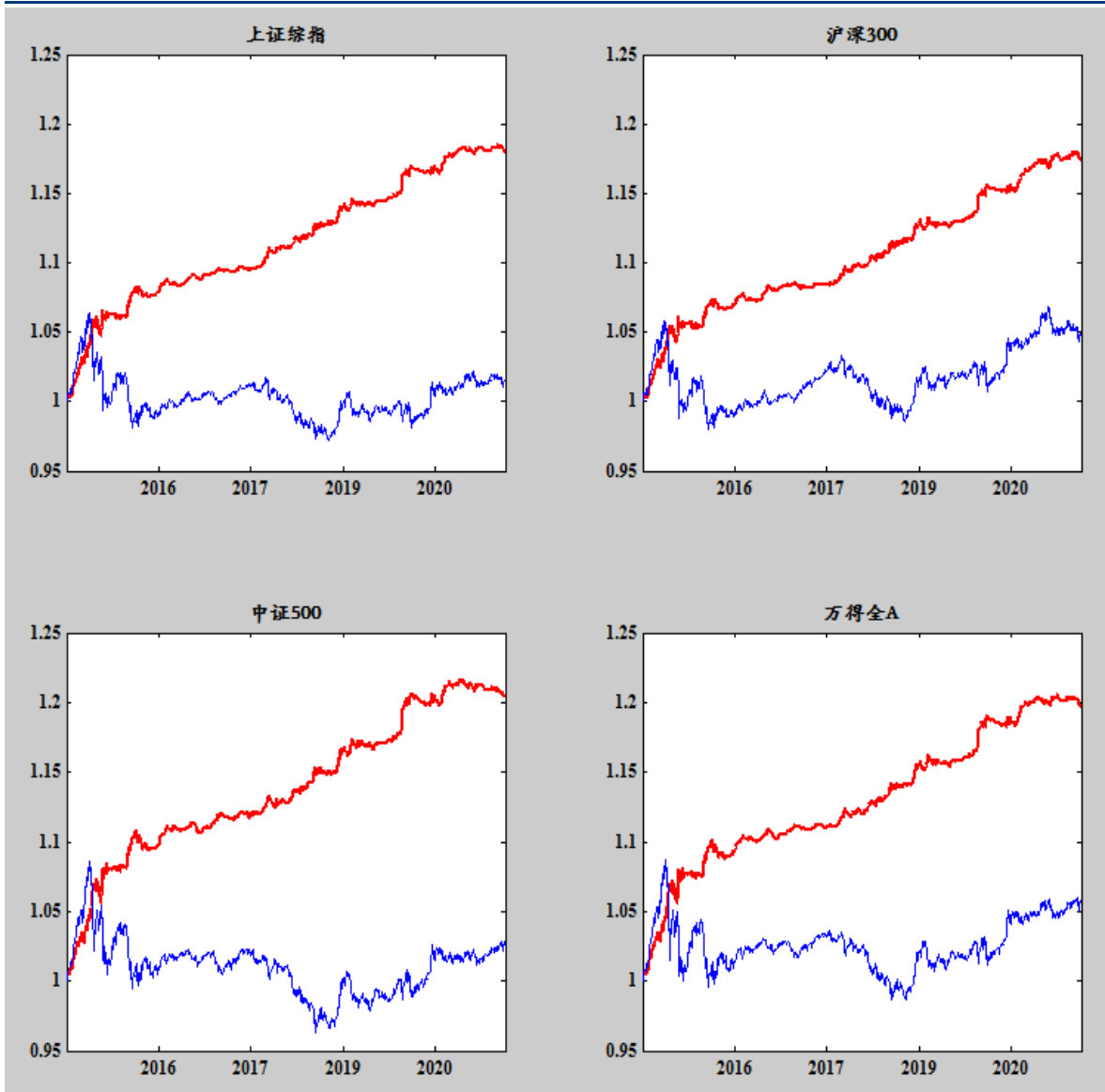
图表 8 综合兵器 V3.2 回测结果(对数图)
