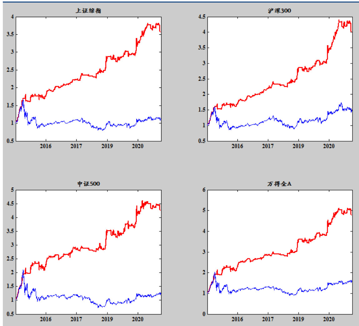
图表 12 综合兵器 V2 做多回测结果
