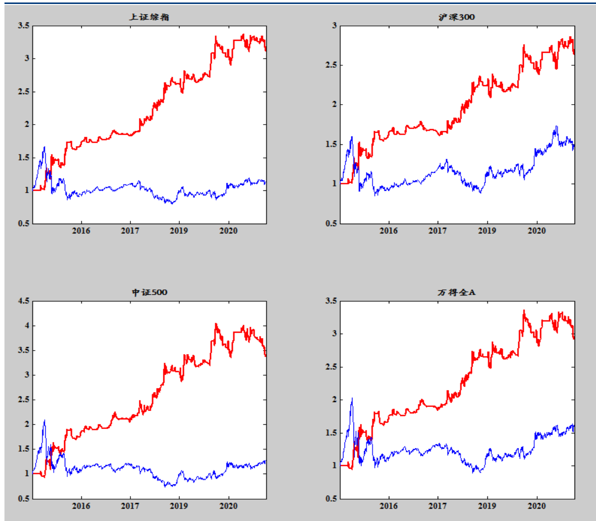
图表 18 综合兵器 V3 做空回测结果
