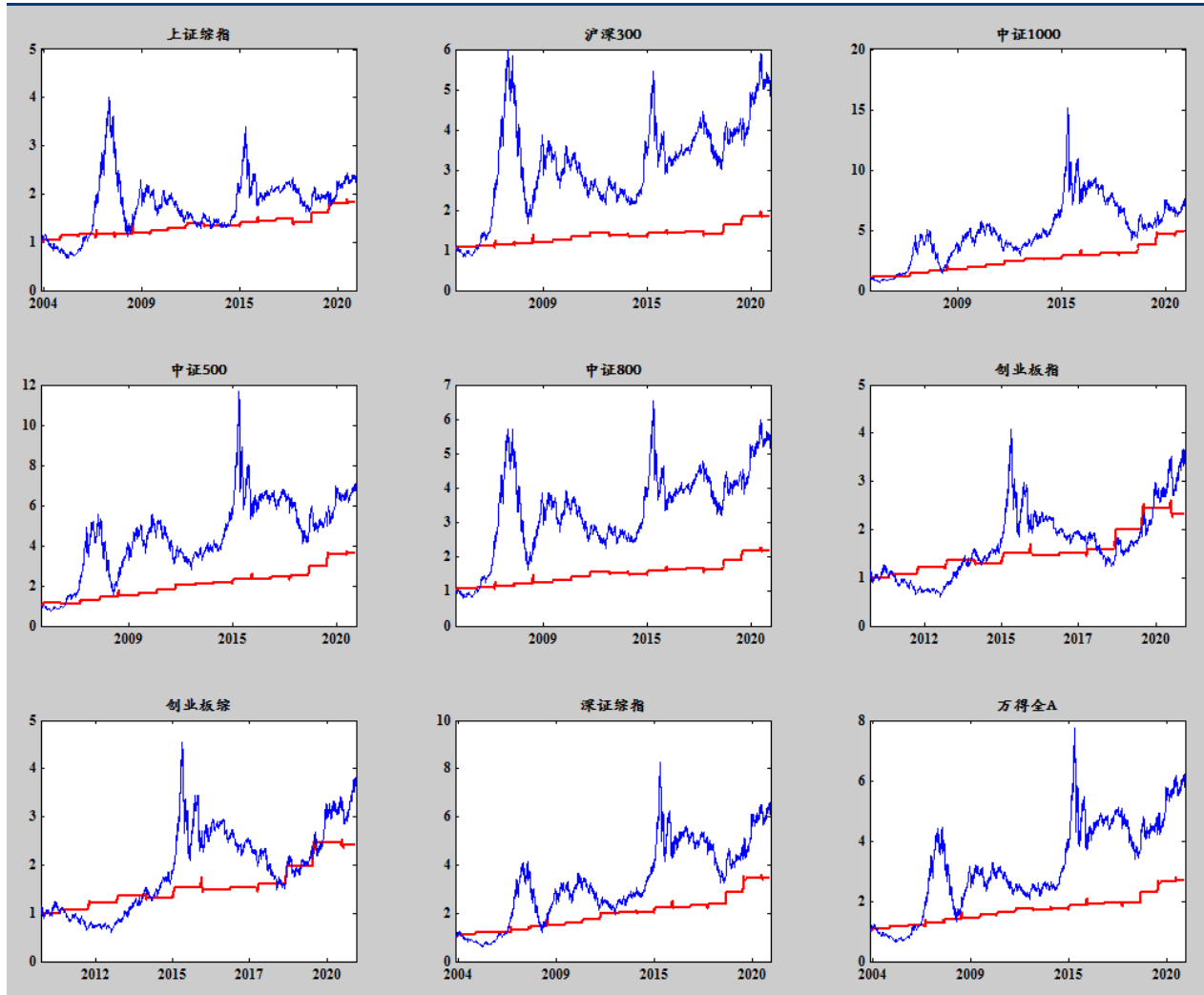
图表 2 增量信息模型择时回测结果
