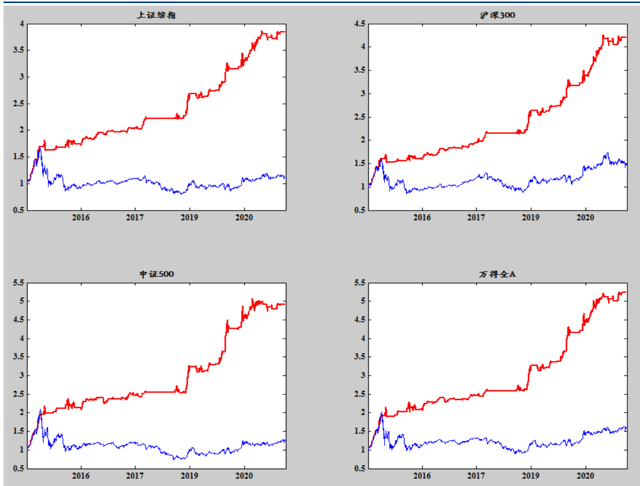
图表 14 综合兵器 V3.2 做多回测结果
