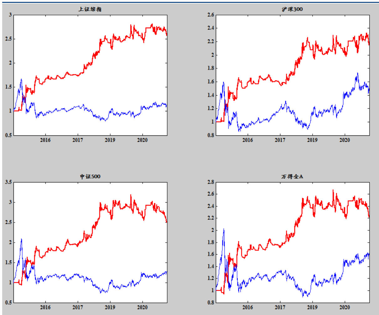
图表 17 综合兵器 V2 做空回测结果
