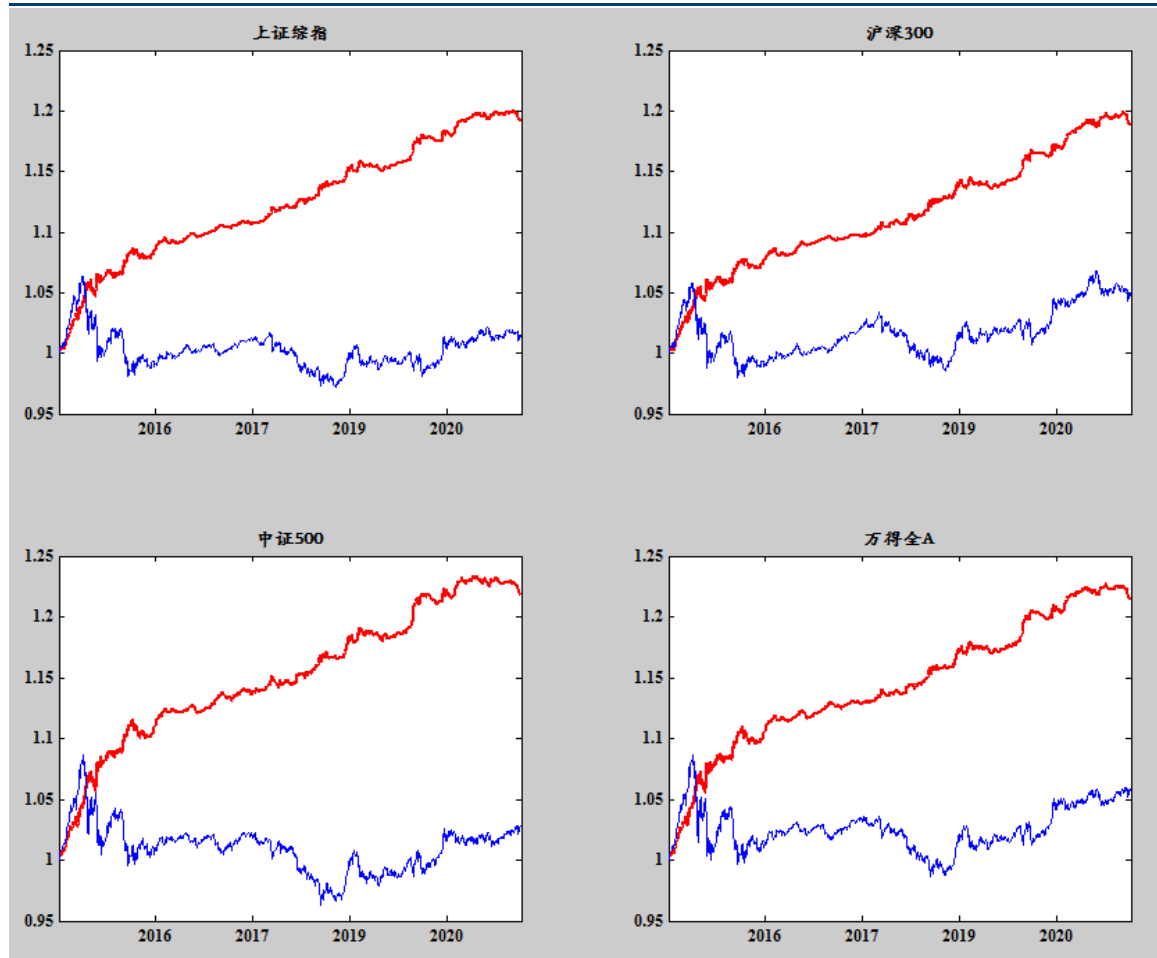
图表 7 综合兵器 V3.1 回测结果(对数图)
