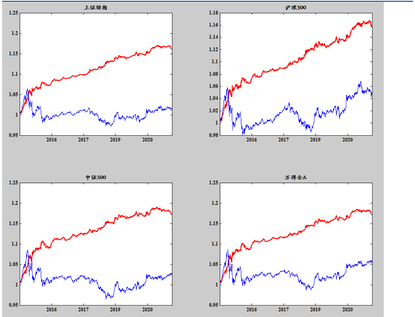
图表 6 综合兵器 V2 回测结果(对数图)
