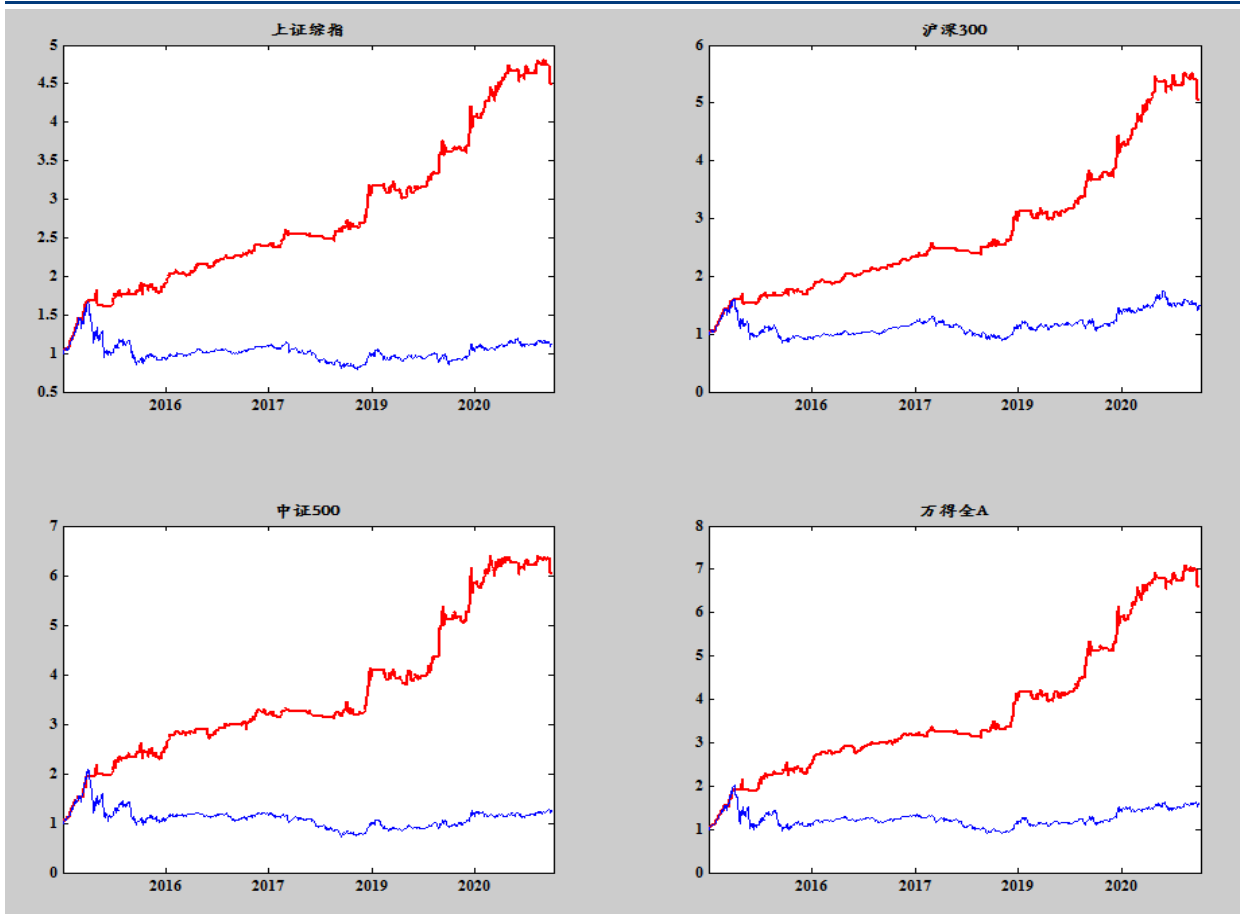
图表 13 综合兵器 V3.1 做多回测结果
