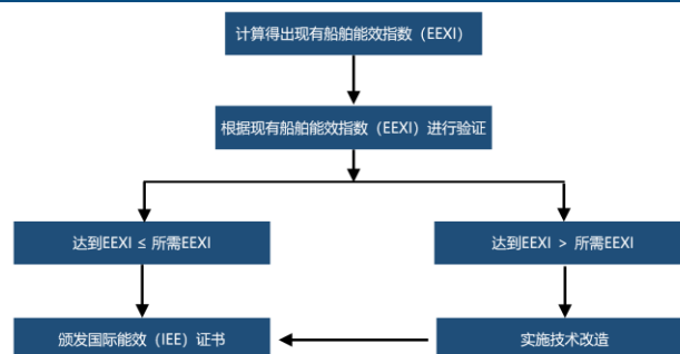
图表39：现有船能效指数 (EEXI) 要求
