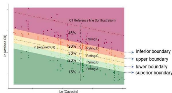
图表41：碳强度评级标准 (CIIT) 每年折减
