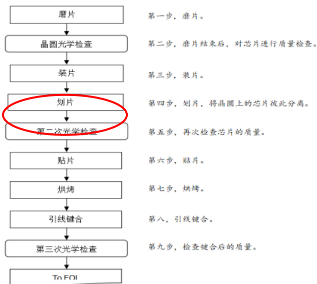
图表 8：半导体晶圆封测前道组装工艺图
