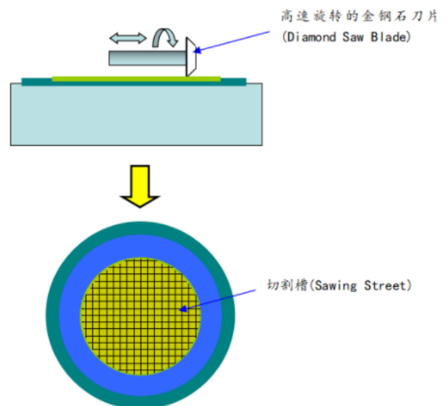
图表 9：封测工序晶片划片工艺示意图
