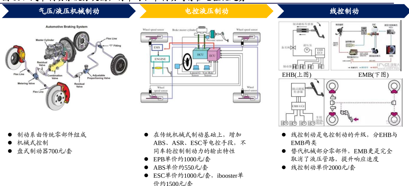
图 39、汽车制动系统分类图，行车与驻车制动均存在电控化趋势
