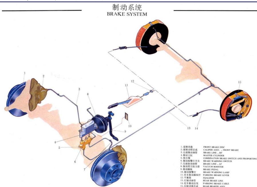
图 22、汽车机械式制动系统结构图
