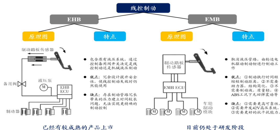
图 42、线控制动 EHB 与 EMB 的特性对比
