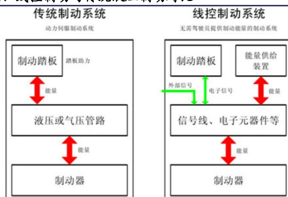
图 41、线控制动与传统液压制动对比
