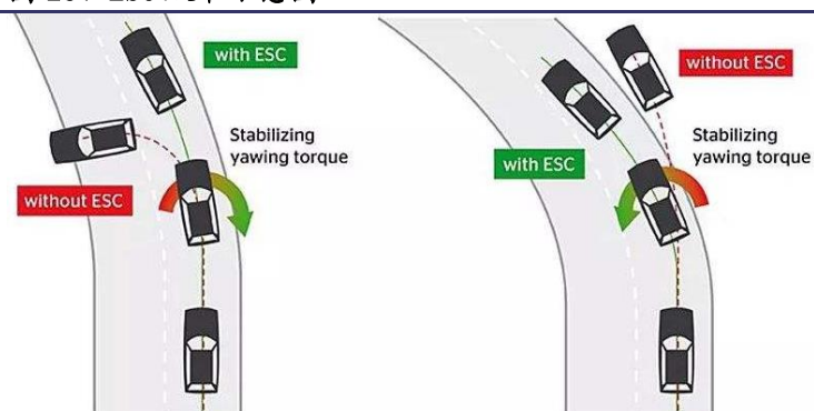
图 25、ESC 效果示意图
