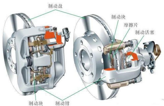
图 17、盘式制动器结构图
