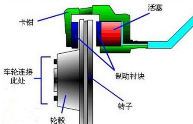
图 18、盘式制动器原理
