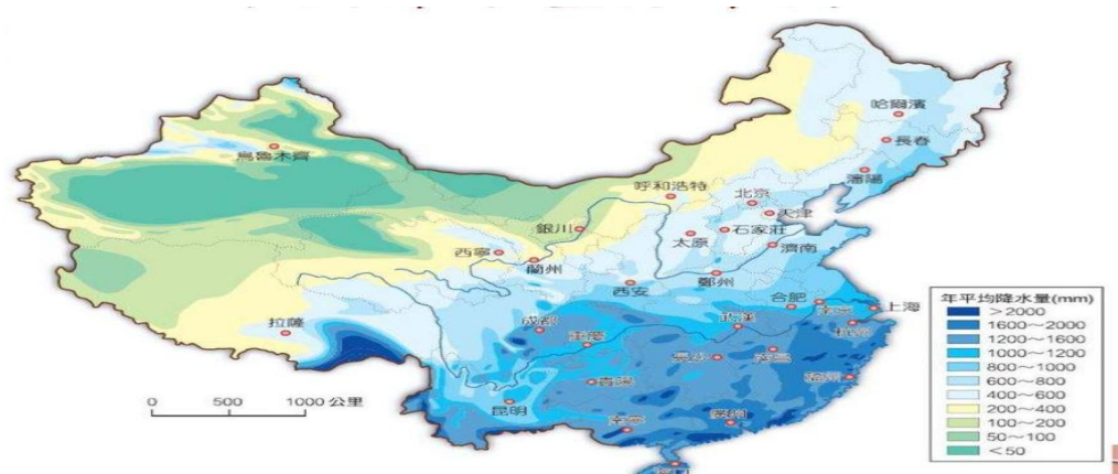
图 19：我国降水量分布图
