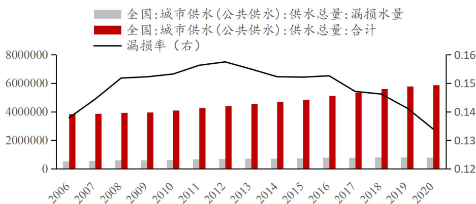
图 22：我国城市供水管网漏损率（万立方米）
