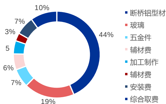
图 7：铝门窗成本拆分
