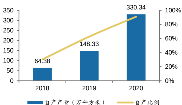
图 29：公司拉丝基布自产情况
