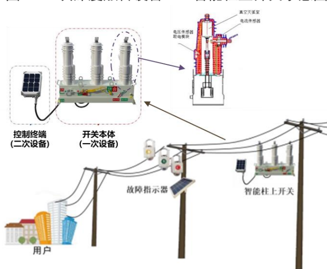
图 一二次深度融合设备——智能柱上开关示意图
