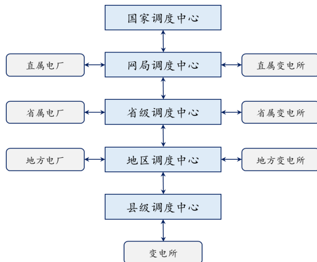
图 调度系统层级结构
