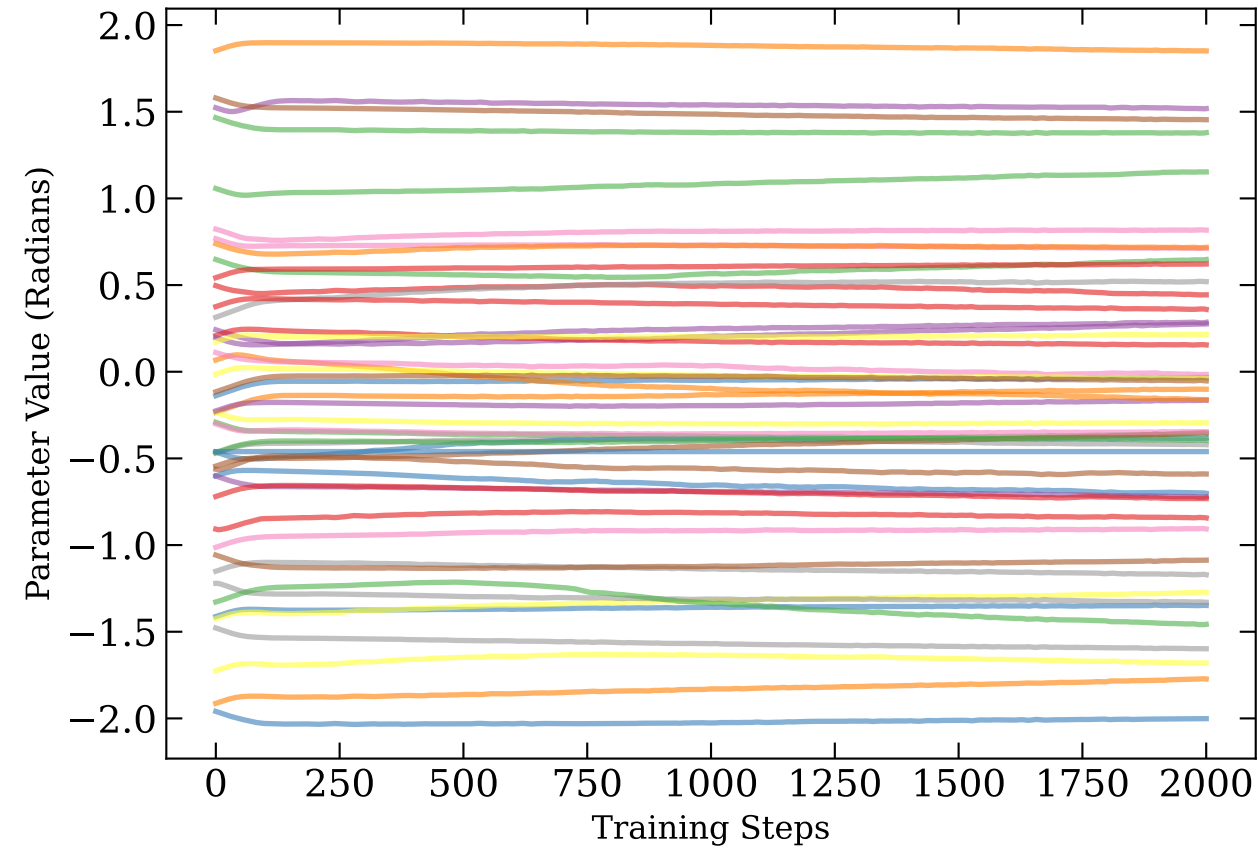
QAE
