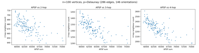
Figure 2: 유향최단 경로 거리 합과 n -홉 도달 쌍 수의 관계 (정점 100개, 간선 286개, 방향 조합 146개). 왼쪽부터 n = 2, 3, 4 .
