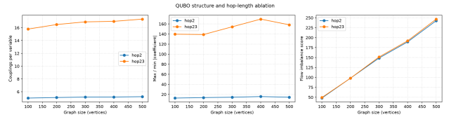
Figure 3: 홉 길이 절제. 왼쪽부터 변수당 커플링 수, 계수 최대·최소 비, 흐름 불균형. hop23은 \lambda_2 = \lambda_3 = 1 , hop2는 \lambda_3 = 0 이다.
