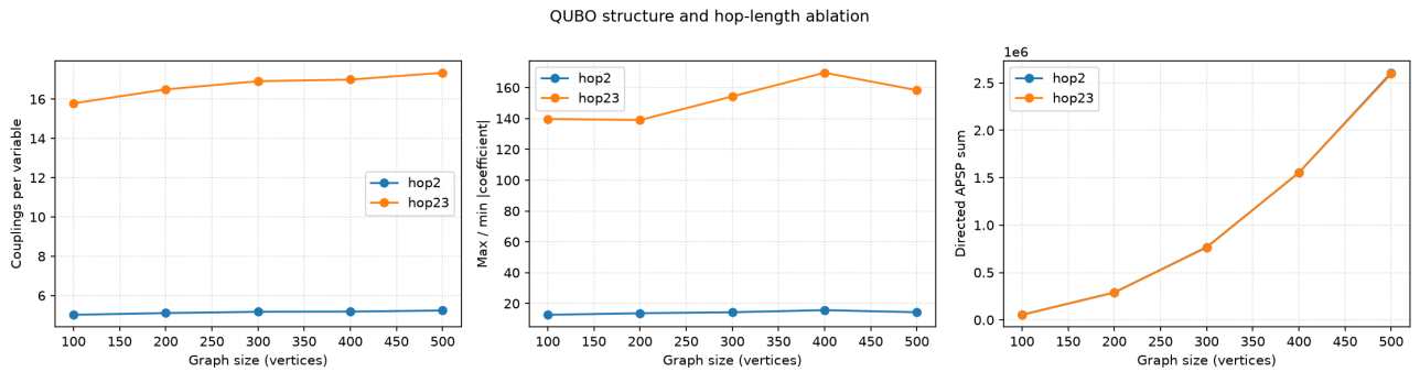
Figure 4: 홉 길이 절제. 왼쪽부터 변수당 커플링 수, 계수 최대·최소 비, 유향 거리 합. hop23은 \lambda_3 = 1 , hop2는 \lambda_3 = 0 이다.
