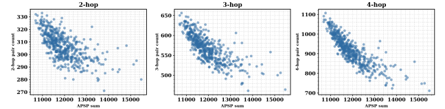
Figure 4: 유향 최단 경로 거리 합과 n -홉 도달 쌍 수의 관계(정점 50개, 간선 137개, 방향 조합 500개). 왼쪽부터 n = 2, 3, 4 .
