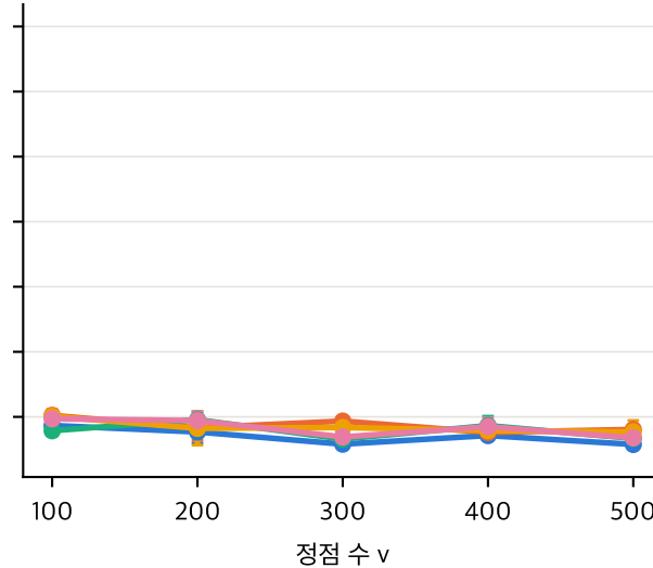
간선 제거 10%
