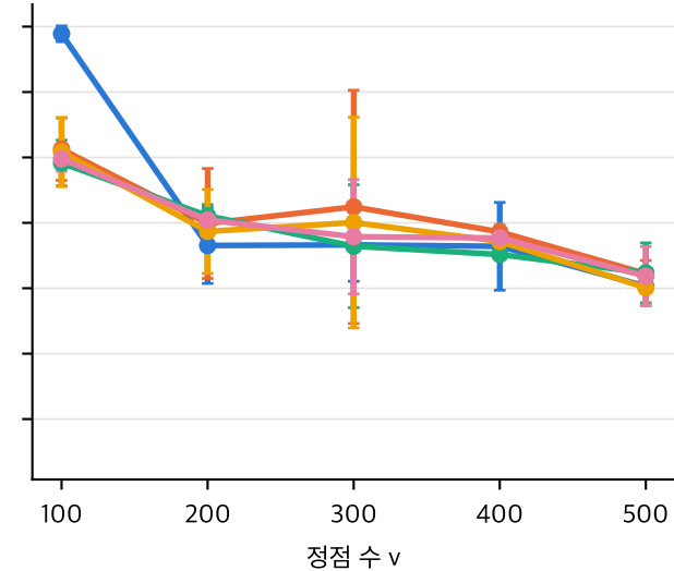
간선 제거 50%
