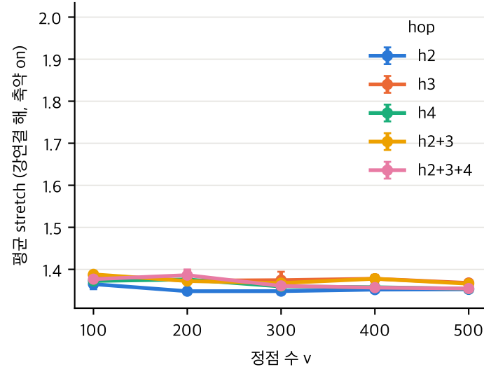
간선 제거 0%
