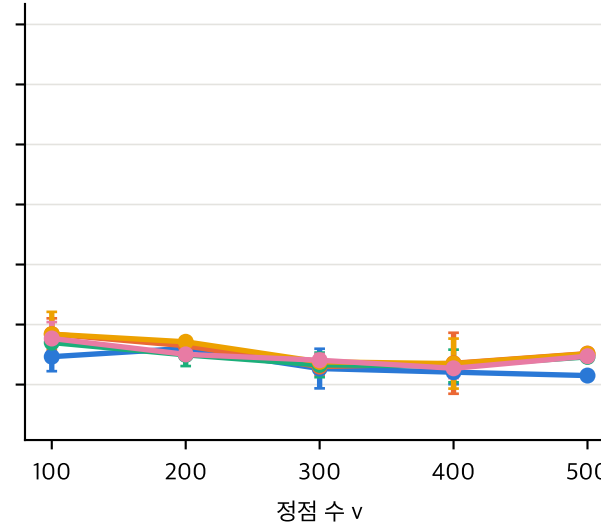
간선 제거 30%
