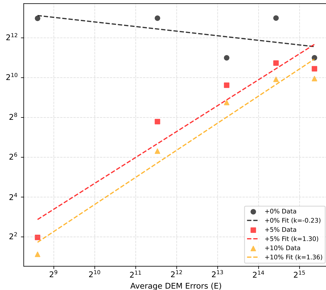
Color Codes
