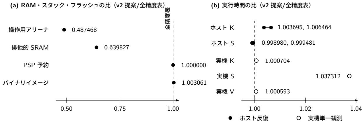
図5 全精度表実装を1としたv2提案実装のRAM、スタック予約、フラッシュ、および実行時間の比。メモリ量はリンク結果と型サイズから得た値である。ホスト計算機上の実行時間は、実行順を反転した二つの30組の測定を別々の点で示す。実機上の実行時間は各一回の観測なので白抜き点とした。測定条件が異なる点は結んでいない。PSP予約量は変わらないが、局所スタックフレームは48-64 bytes増加した。
