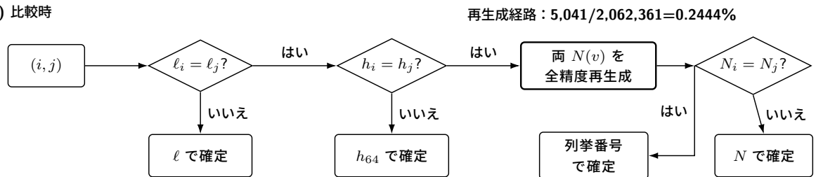
図3 ノルム要約の保存形式と比較経路。ビット長または上位 64 bit が異なる場合は、要約だけで比較結果が決まる。両者が一致した場合は、圧縮候補から全精度ノルムを再生成する。図中の再生成率は固定鍵実行時間検査で観測した値であり、比較結果の正しさはこの頻度に依存しない。
