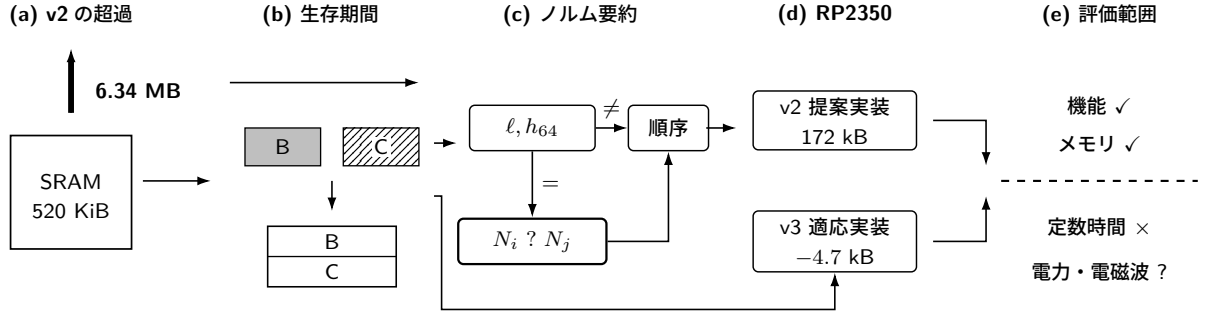
図1 本研究の全体像。v2 提案実装では生存期間配置とノルム要約を組み合わせる。v3 適応実装では、生存期間配置を格子簡約と署名処理の二つの関数へ転用する。両実装を RP2350 上で評価し、機能・メモリの評価とサイドチャネル評価を分けて示す。
