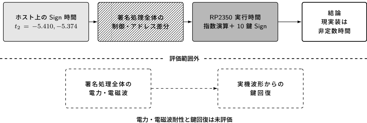
図6 サイドチャネル評価の範囲。実線枠は本研究で得た検出結果、破線枠は実施していない実験を表す。現実装の変時間性は検出したが、署名処理全体の電力・電磁波への耐性や、鍵を回復できるかどうかは判定していない。
