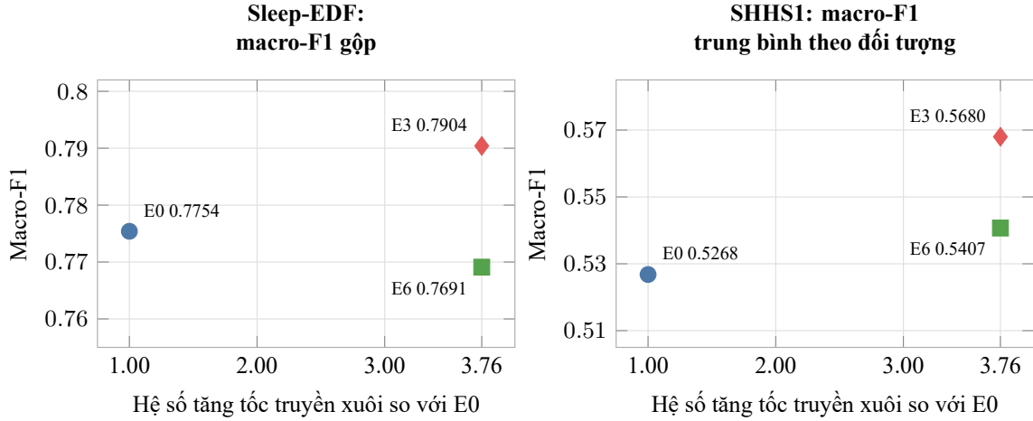
Hình 2. Hệ số tăng tốc truyền xuôi đo được và macro-F1 tổng hợp của các cấu hình chính seed 42. Chỉ biểu diễn E0, E3 và E6. Ở bên trái báo cáo macro-F1 gộp trên Sleep-EDF; ở bên phải báo cáo macro-F1 trung bình theo đối tượng trên mẫu SHHS1. Hệ số tăng tốc được tính so với E0 trong benchmark truyền xuôi cố định. Biểu đồ được tạo từ kết quả tổng hợp đã lưu bằng mã PGFPlots có thể chỉnh sửa; OpenAI Codex hỗ trợ viết mã vẽ.
