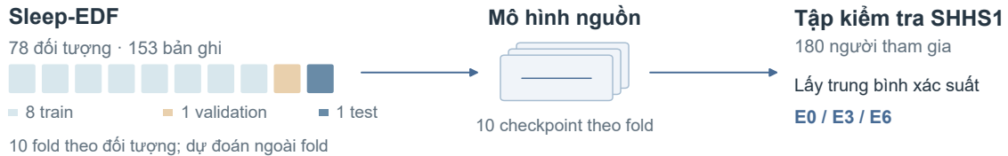
Hình 1. Các cấu hình mô hình và quy trình đánh giá. (a) E0 và E1 dùng chung bộ mã hóa 15-CNN: năm nhánh cho mỗi epoch hiện tại, liền trước và liền sau tạo thành 75 đặc trưng cho BiLSTM hoặc TCN. E2, E3, E4 và E6 dùng bộ mã hóa ResNet-1D cho epoch hiện tại, được huấn luyện riêng theo từng cấu hình, cùng TCN. Các số trong ResNet biểu thị số kênh đầu ra; GAP là phép lấy trung bình toàn cục. Cả hai TCN đều có sáu khối tích chập giãn không nhân quả. E3 và E6 còn cắt biên độ tại \pm 800 \mu V sau lọc thông dải; E3 chia cho 100, còn E6 dùng thống kê z-score của toàn bản ghi. (b) Sleep-EDF dùng mười fold theo đối tượng, chung cho các cấu hình; mỗi lượt gồm tám fold huấn luyện, một fold xác thực và một fold kiểm tra. Đánh giá chính trên SHHS1 so sánh E0, E3 và E6 trên 180 người tham gia, lấy trung bình xác suất từng lớp từ mười checkpoint nguồn trước khi chọn lớp dự đoán, không huấn luyện mô hình trên miền đích. E6 dùng thống kê bản ghi đích không nhân. E5 chỉ kiểm tra tính đồng nhất của đầu vào, không phải một cấu hình đánh giá hiệu năng bổ sung. Thiết lập huấn luyện và các phân tích bổ sung được mô tả trong phần Phương pháp và tài liệu bổ sung. Sơ đồ được vẽ bằng Matplotlib với sự hỗ trợ của OpenAI Codex; các ký hiệu biểu diễn cấu trúc mô hình và vai trò của fold, không phải tín hiệu đo hay kích thước phân hoạch.
