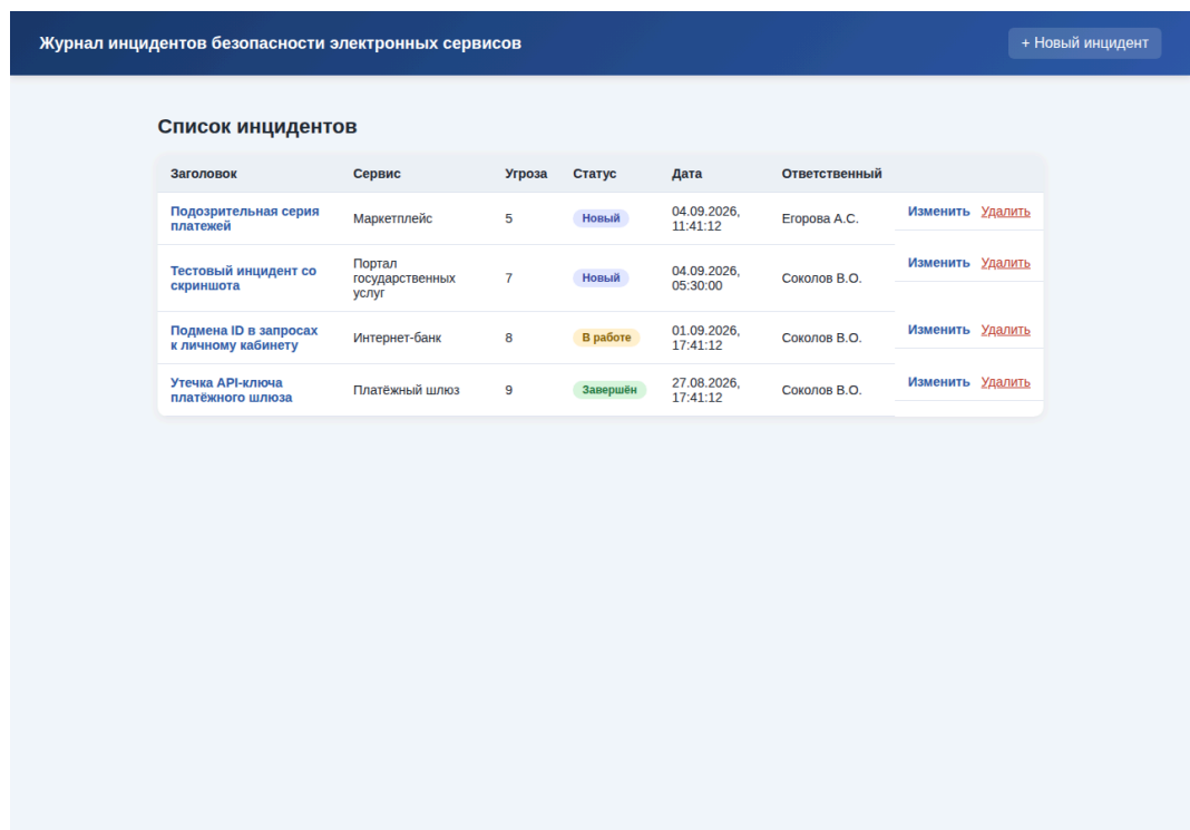
Рисунок 6 — главная страница со списком, включающим новый инцидент
