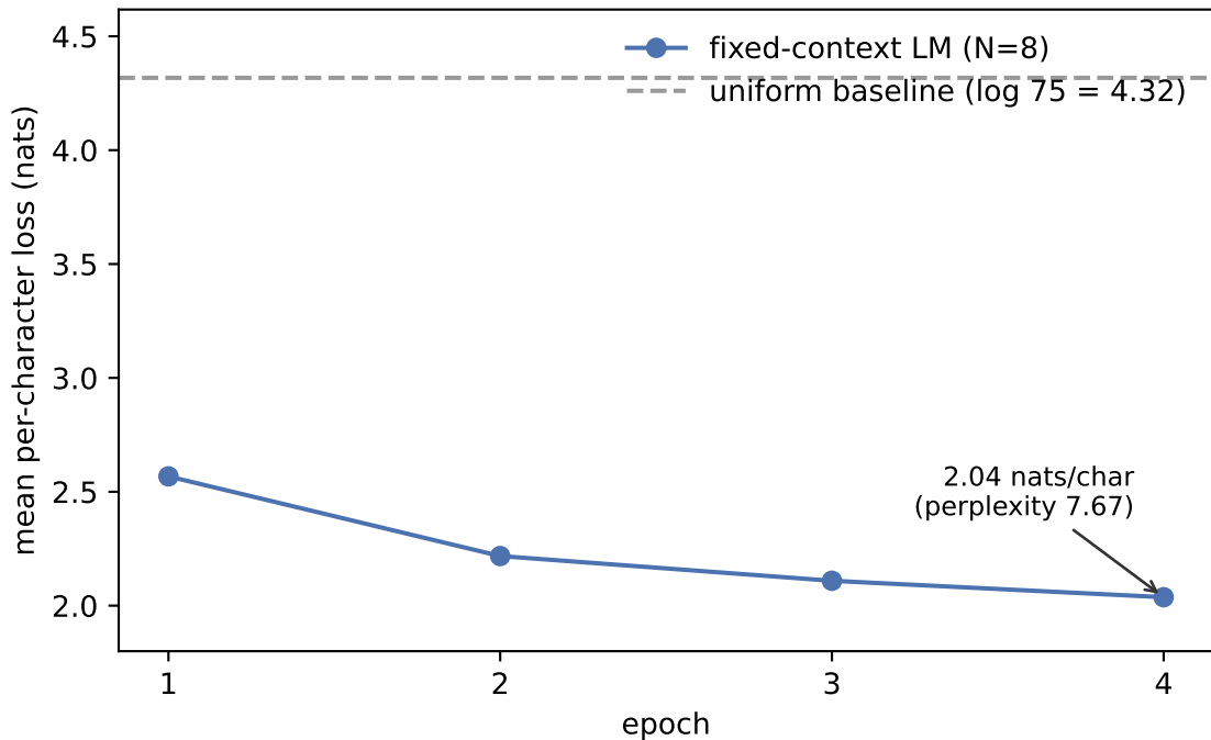
Char-level Alice: loss per epoch
