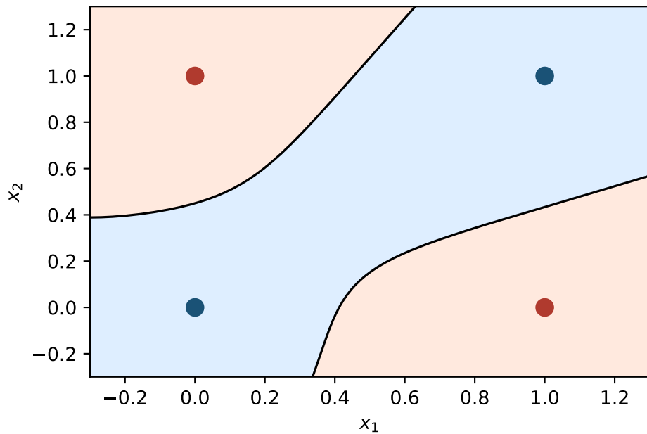
MLP 2-8-1 Tanh
