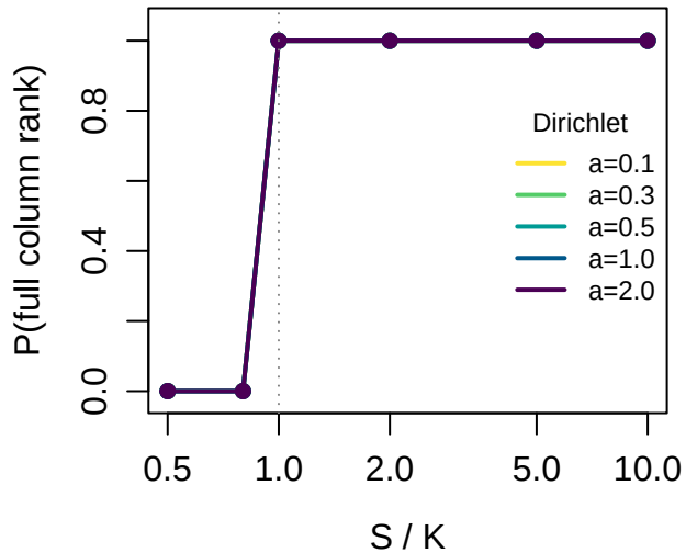
A. Rank condition ( K=10 )
