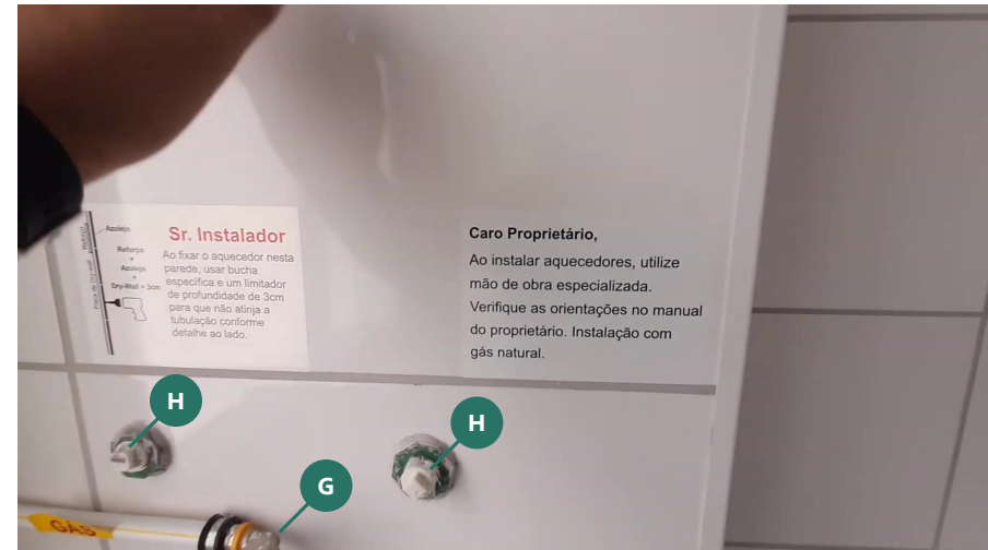
AD-0278 • L-H02: conexões • L-G01: gás • aviso do aquecedor
