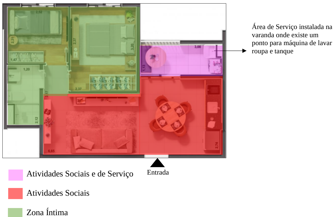
Figura 43 - Planta Bipartida de um apartamento com 40,77 m 2
