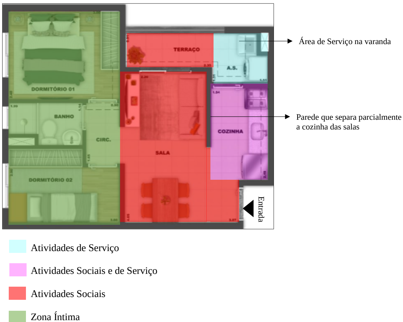
Figura 37 - Planta Parcialmente Integrada de um apartamento com 40,13 m 2
