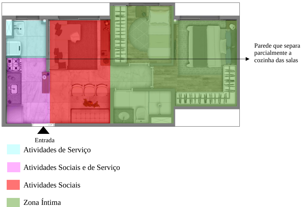
Figura 36 – Planta Parcialmente Integrada de um apartamento com 38 m 2
