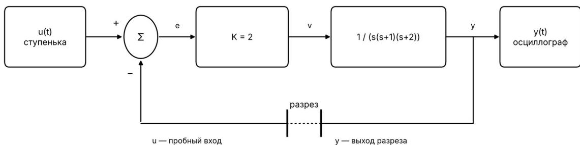
Рисунок 3 – Размыкание контура: связь удаляется, в разрез подаётся пробный вход u , а выход y измеряется
