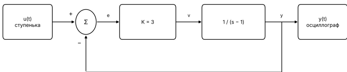
Рисунок 1 – Замкнутая система с отрицательной обратной связью
