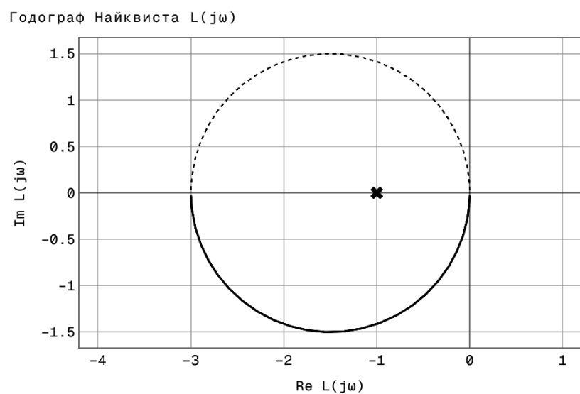
Рисунок 5 – Годограф Найквиста для неустойчивого объекта 3/(s - 1) : окружность охватывает точку -1
